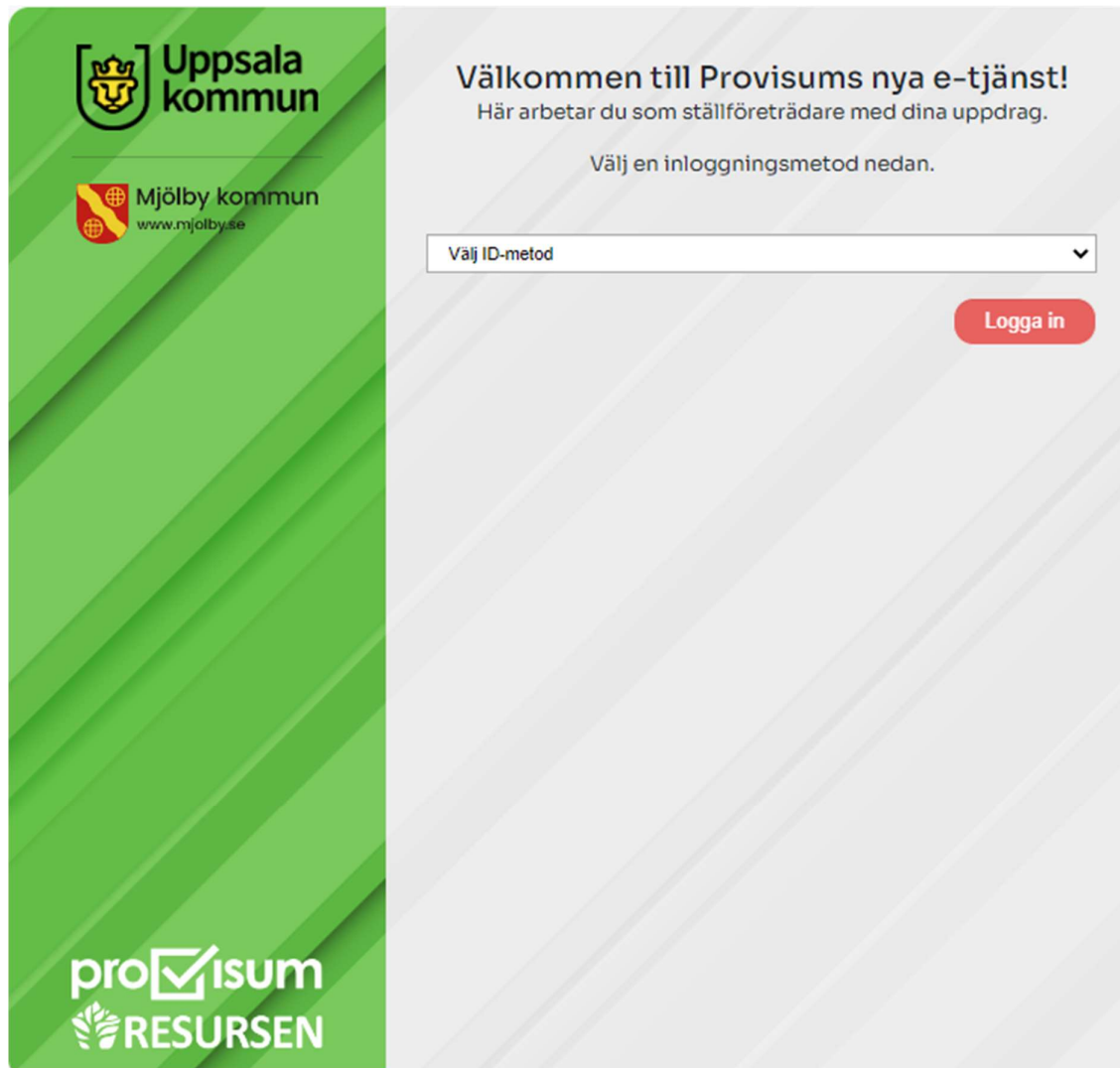
Figur 1: Inloggningsvy
